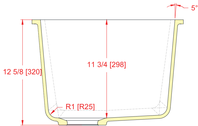
Section A-A DuPont 5216
